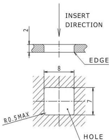
安装孔形状 (参考)
